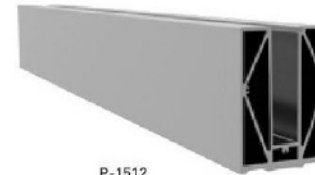
P-1512 7,53 Kg/m
