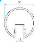
P-AL5148 1,270 Kg/m On-Glass Profile Handläufe De Profiles sur verre
