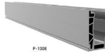
P-1008 5,852 kg/m
