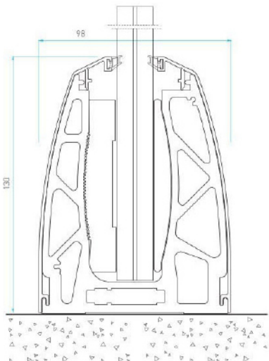
C70-8401
